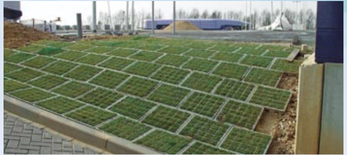
TTE® direct green Elemente für die Hangsicherung, auch ideal für die Dachbegrünung.
